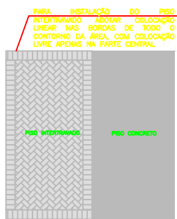
DETALHE BORDA PISO INTERTRAVADO SEM ESCALA
