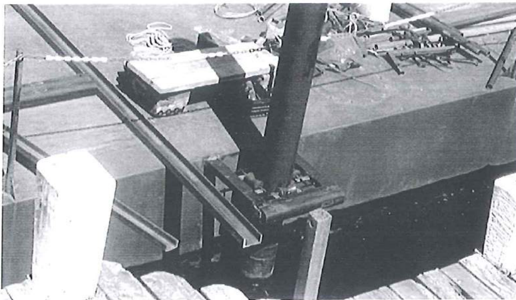
Figura 9 – Modelo de travamento proposto, constituído por estacas e roletes que permitem a oscilação vertical do flutuante.
